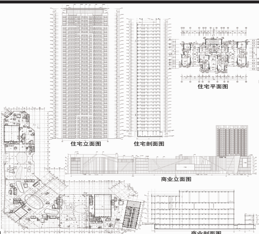
商业剖面图
