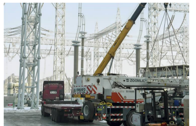
昌吉—古泉±1100千伏特高压直流输电工程途经新疆、甘肃、宁夏、陕西、河南、安徽六省区。工程满负荷投运后,每年可向华东地区输送电量660亿千瓦时。目前,昌吉—古泉±1100千伏特高压直流输电工程建设进入尾声,预计12月底完工。届时,该工程将具备全面投运条件。图为昌吉换流站施工现场。(新华网)
