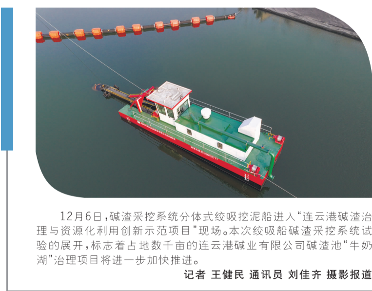
12月6日,碱渣采控系统分体式绞吸挖泥船进入“连云港碱渣治理与资源化利用创新示范项目”现场。本次绞吸船碱渣采控系统试验的展开,标志着占地数千亩的连云港碱业有限公司碱渣池“牛奶湖”治理项目将进一步加快推进。
