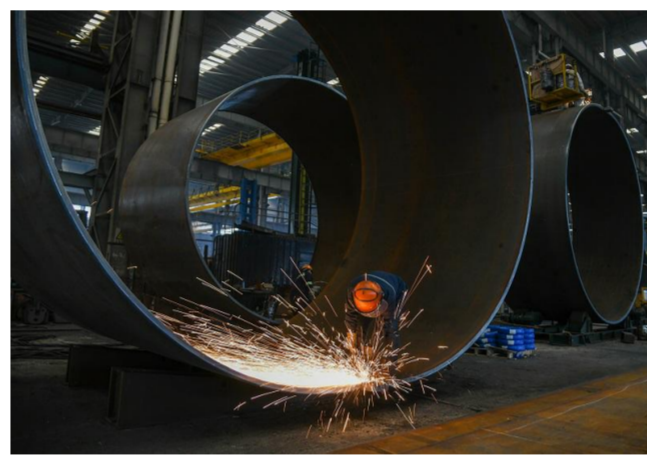
江苏长风海洋装备制造有限公司工人正在焊接海上风电钢管桩。
