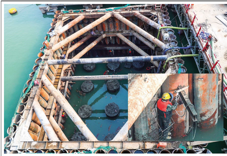
总投资约4.45亿元的淮河大桥改造工程全长2063米,目前大桥的桩基建设基本完成。因为工人在主桥墩浇筑关键处精心施工。 融媒体记者 许昌银振
