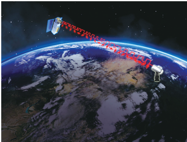
这是量子微纳卫星“济南一号”星地量子密钥分发实验示意图。
